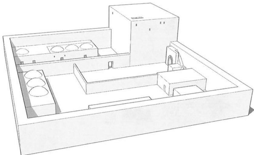
Afb. 4: Reconstructie van een groot ommuurd complex (M.Hense).
