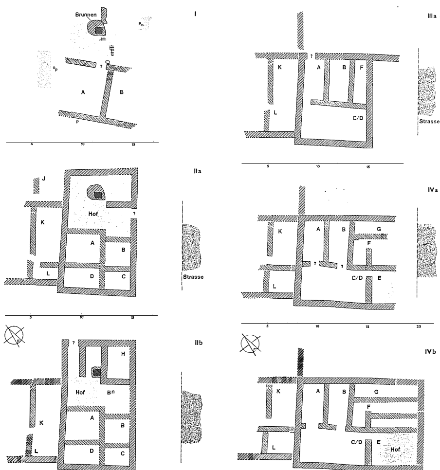
Fig. 3 — Reconstructie-plattegronden van de huizen in de Hamburgse opgraving, archaïsche fasen I-IV; stand 1991 (naar Vorbericht I , 204 fig. 2-3).
