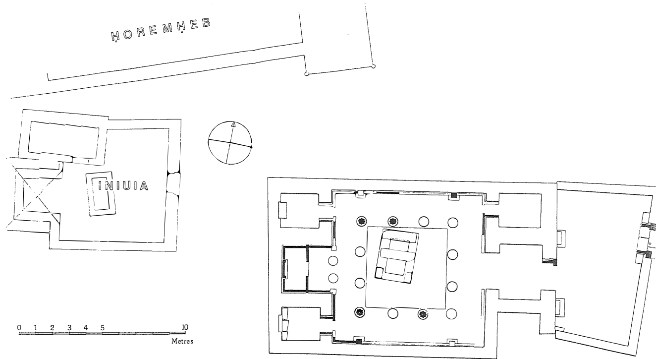
Plattegrond van het grafcomplex van Pay en Raia. De op de wanden bewaard gebleven reliëfs zijn aangeduid in zwart.
