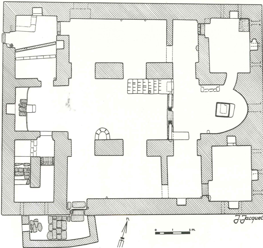
Fig. 66. Plattegrond van de kerk van Abdallah Nirqi.
