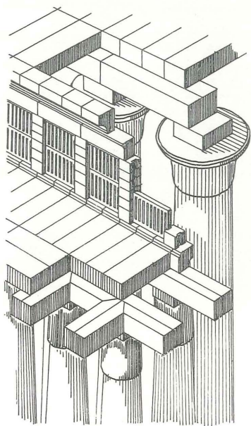
Fig. 77. Schets van de dakconstructie van een hypostyle zaal.
